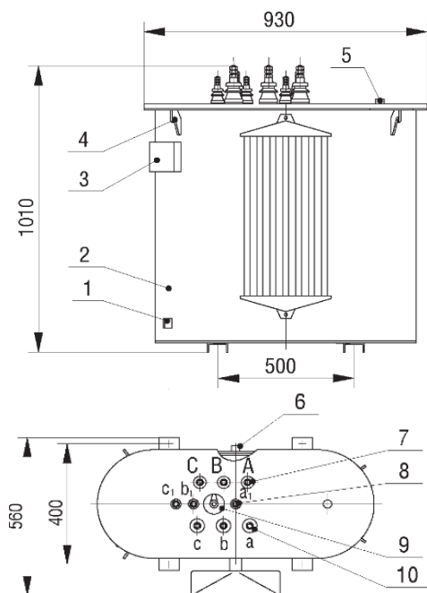
ТМТО-80/0,38-У1
