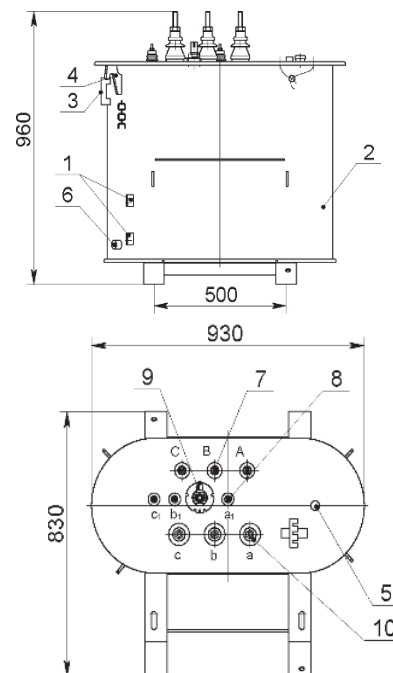
ТМТО-50/0,38-У1
